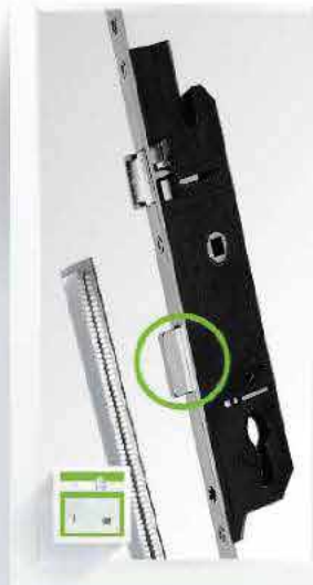
K1062 Kesilebilir Kilitli Kapı İspanyolet (Dilsiz) Boylar : 170-220cm
