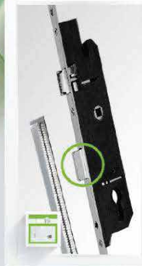
K1056 Kesilebilir Kilitli Kapı İspanyolet (Dilsiz) Boylar : 170-220cm
