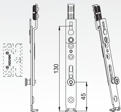
İspanyolet Ek Parça Se, 90°
