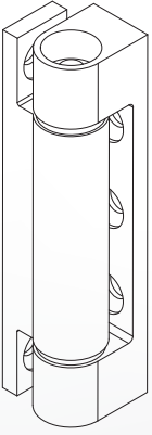
Menteşe 75 mm
