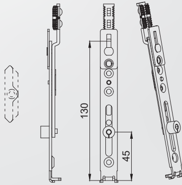
İspanyolet Ek Parça, 180°
