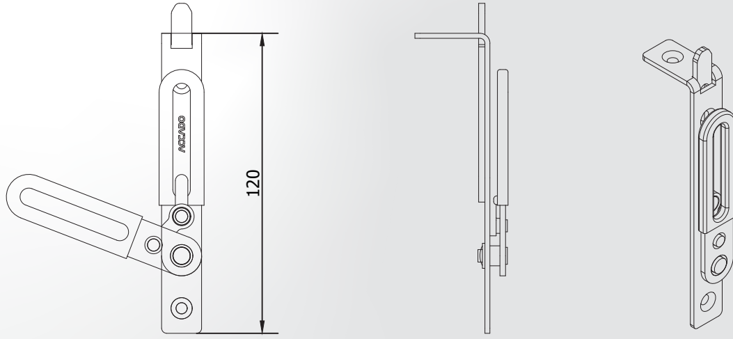
Levyeli Fişek Sürgü Alt/Üst 120 mm
