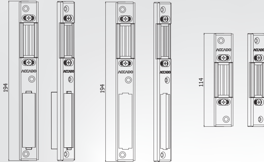
Ayarlı Kapı Kilit Karşılığı Eko Sürgü Plastikli
