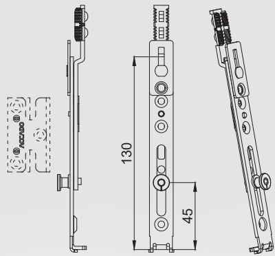
İspanyolet Ek Parça Se, 180°
