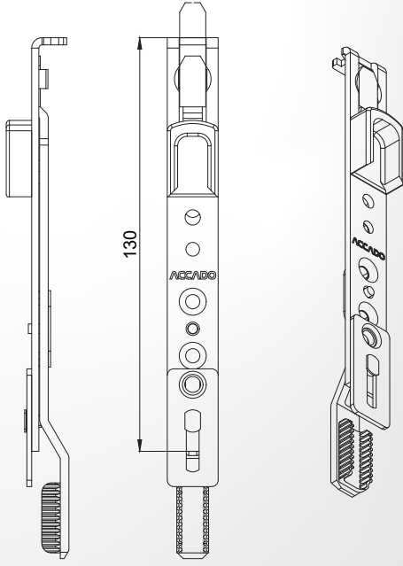
Üst Fişek Sürğü
