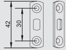
Sürme İspanyolet Merkezleme Parçası
