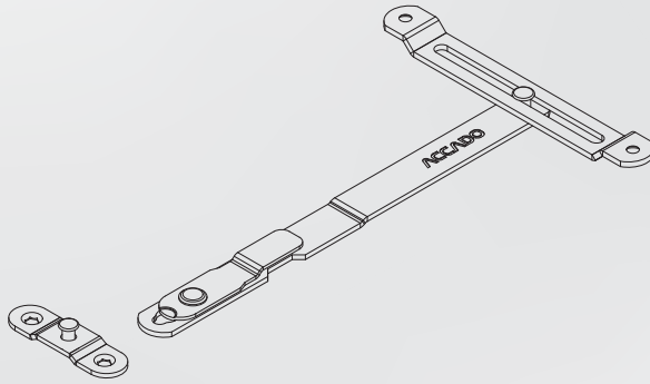
Bağlantılı Vasistas Makas Kanat Parçası
