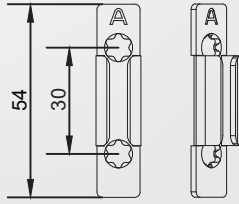
Sürme İspanyolet Karşılığı - Sac
