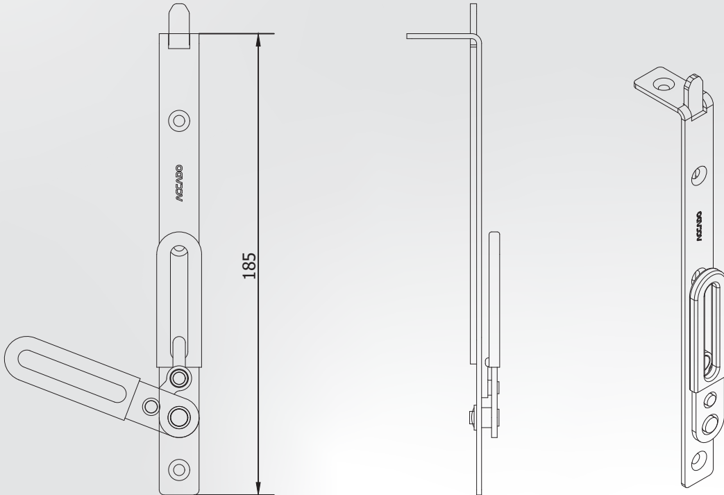
Levyeli Fişek Sürgü Alt/Üst 185 mm
