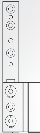
Ayarlı Alt Mentefe
