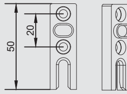
Sürme İspanyolet Karşılığı - Zamak
