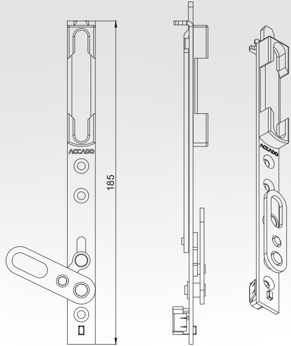
Levveli Alt Fişek Sürğü
