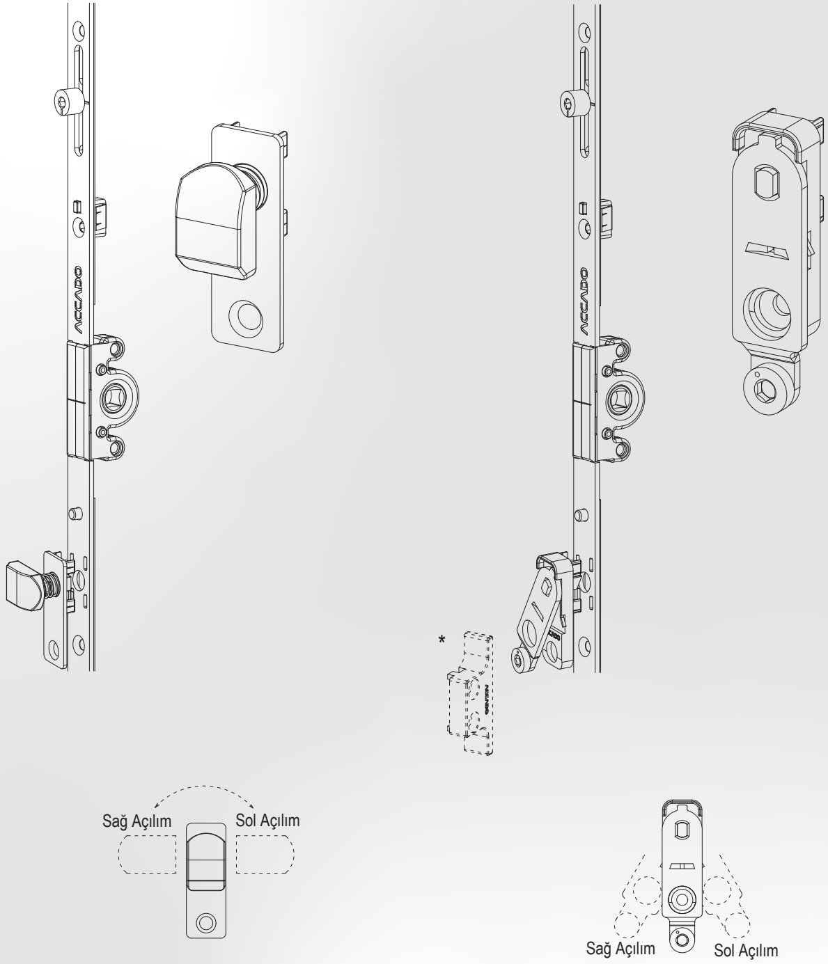
Devrilme Emniyeti (karşılık kullanılmaz)
