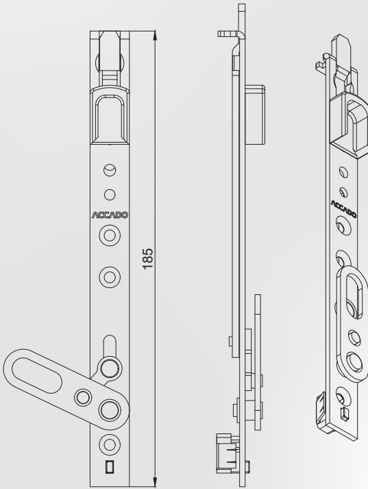
Levveli Üst Fişek Sürğü
