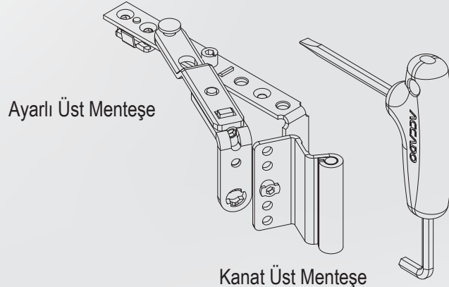
Tek Açılım Uygulaması
