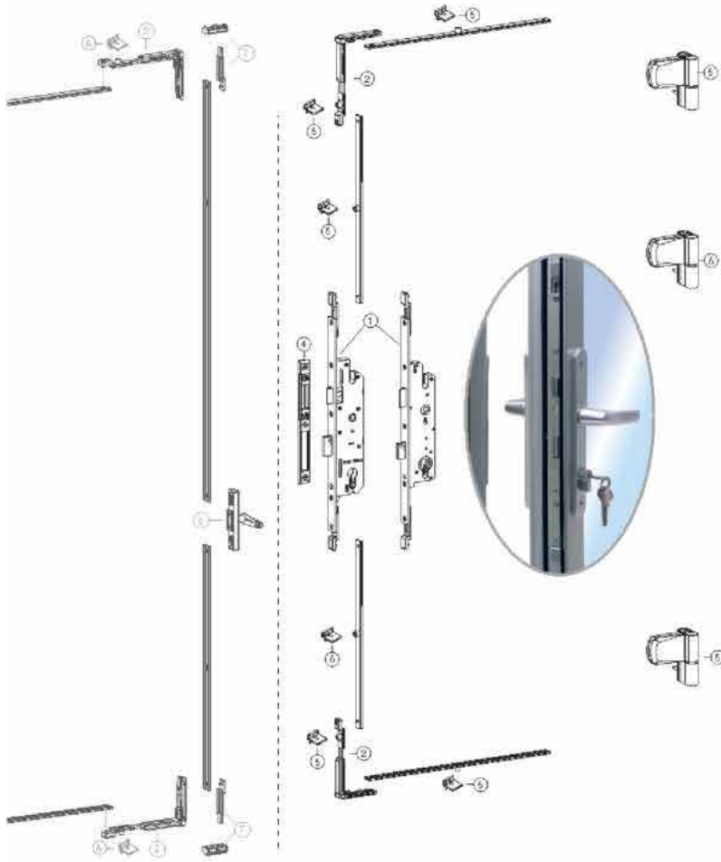
Koldan Kumandalı Çalıştırma Şekli
