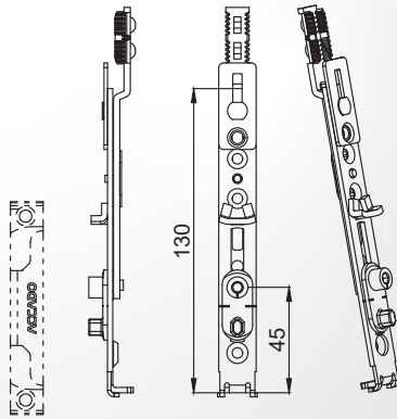
Bottom Extension-1, 420-950
